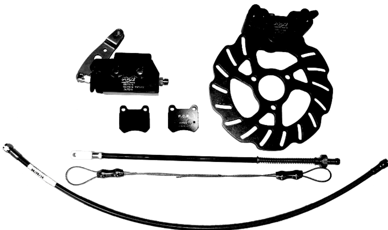
FOTO DEL SISTEMA FRENANTE COMPLETO PRESENTATO ALL'ATTO DELL'OMOLOGAZIONE
