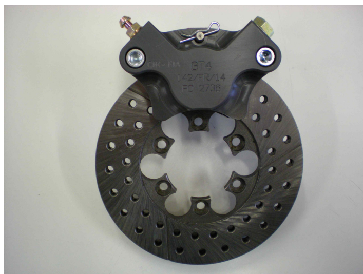
Photo du frein avant : étriers et disques seulement Photo of front brake: calipers and discs only
