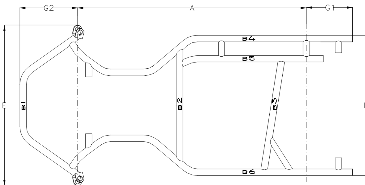
VUE DE DESSUS / VIEW FROM ABOVE
